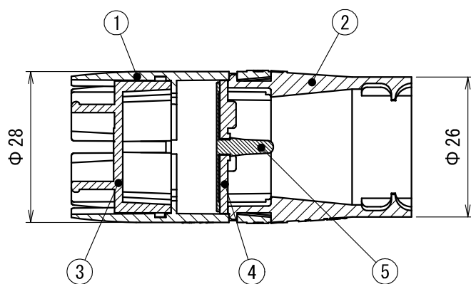
断面 A-A
